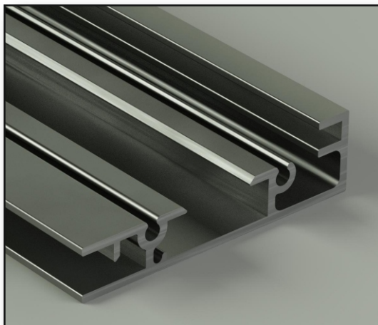
MOD1 Perfil Modular abierto.
