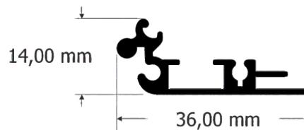
AB02 Perfil Base de marco abatible.
