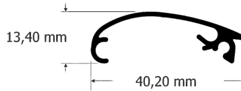
AB01 Perfil Tapa de marco abatible.
