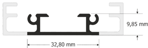
MOD3 Perfil Modular de refuerzo.
