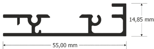
MOD1 Perfil Modular abierto.
